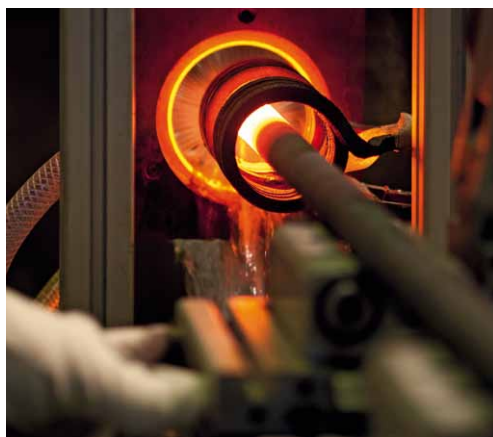
Индуктивная закалка зубил Inductive tempering
