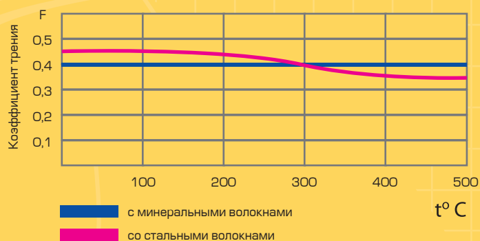
Зависимость коэффициента трения от t° C на поверхности тормозного диска
