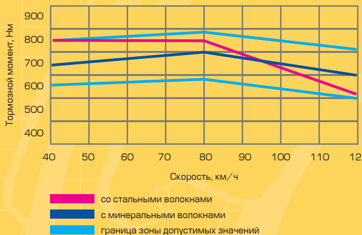
Зависимость тормозного момента от скорости движения автомобиля
